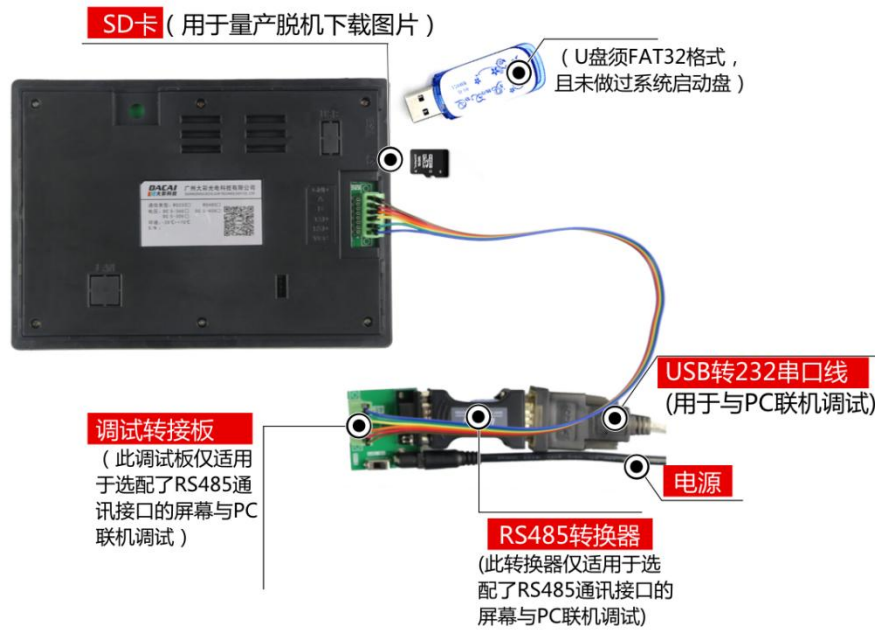
图 1-4 RS485 调试工具图
